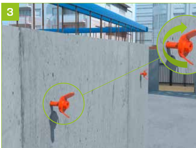
3 - Un écrou papillon est vissé de l'autre côté du voile pour serrer et bloquer chaque clap.
