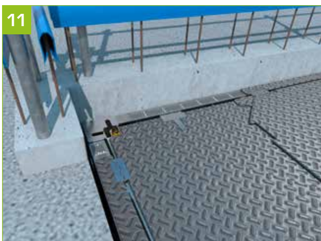
- Les crochets de levage se rétractent et les tôles se rabattent automatiquement.
